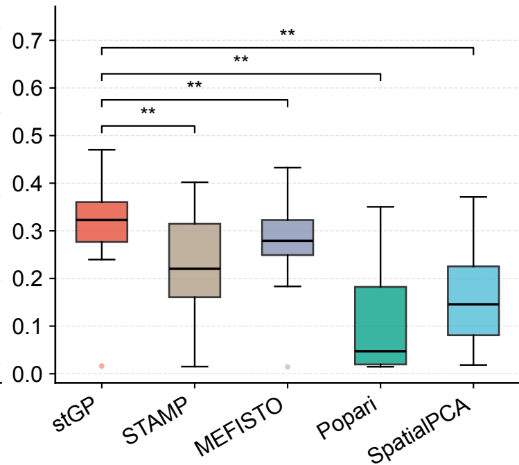
NMI
